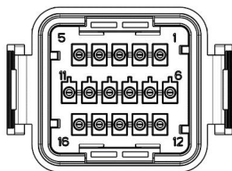
图 5.7 DRM &amp; CT 端子正视图
