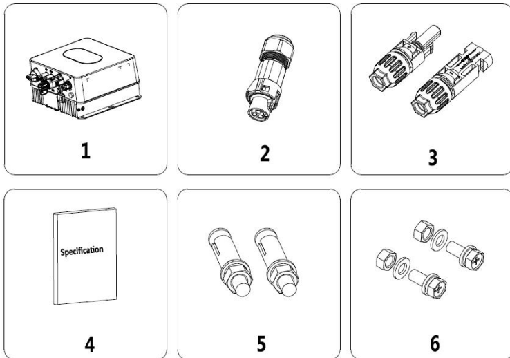
图 4.1 单相逆变器 XG1-5KTL-S 交付内容
