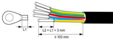
图 5.6 压接电缆端子
