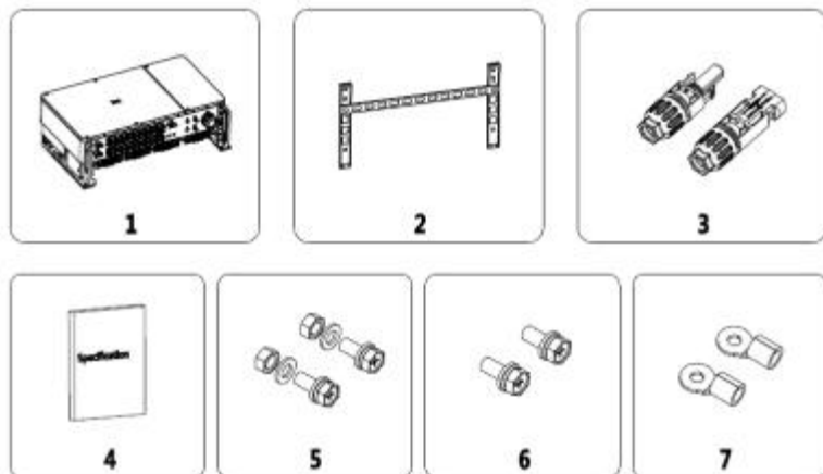
图 4.1 三相逆变器 100-136kW 交付内容
