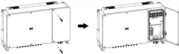
图 5.5 拆开机器面盖
