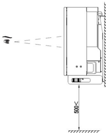
图 4.3 最佳安装高度区域
