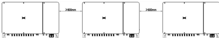
图 4.5 并排安装尺寸要求
