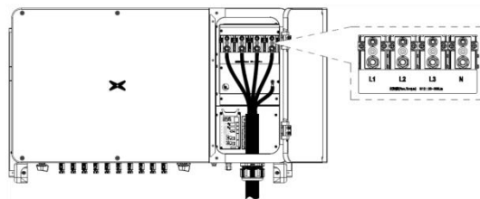
图 5.7 三相逆变器电网接入
