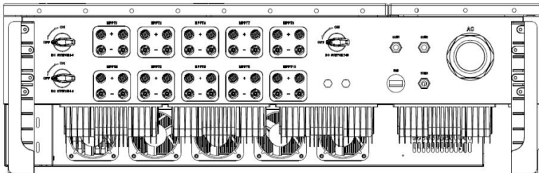
XG110TR 底部视图
