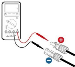
图 5.3 测量直流输入电压
