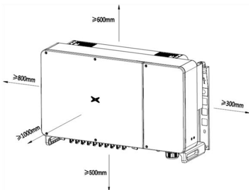
图 4.4 逆变器安装间距
